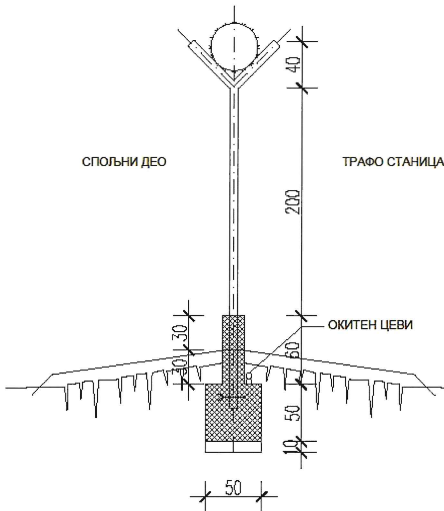
Сл. 9 Попречни профил ограде око трафо станице
